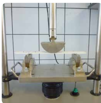
Prüfanordnung für die S1/S2-Prüfung gemäß DIN EN 12004
